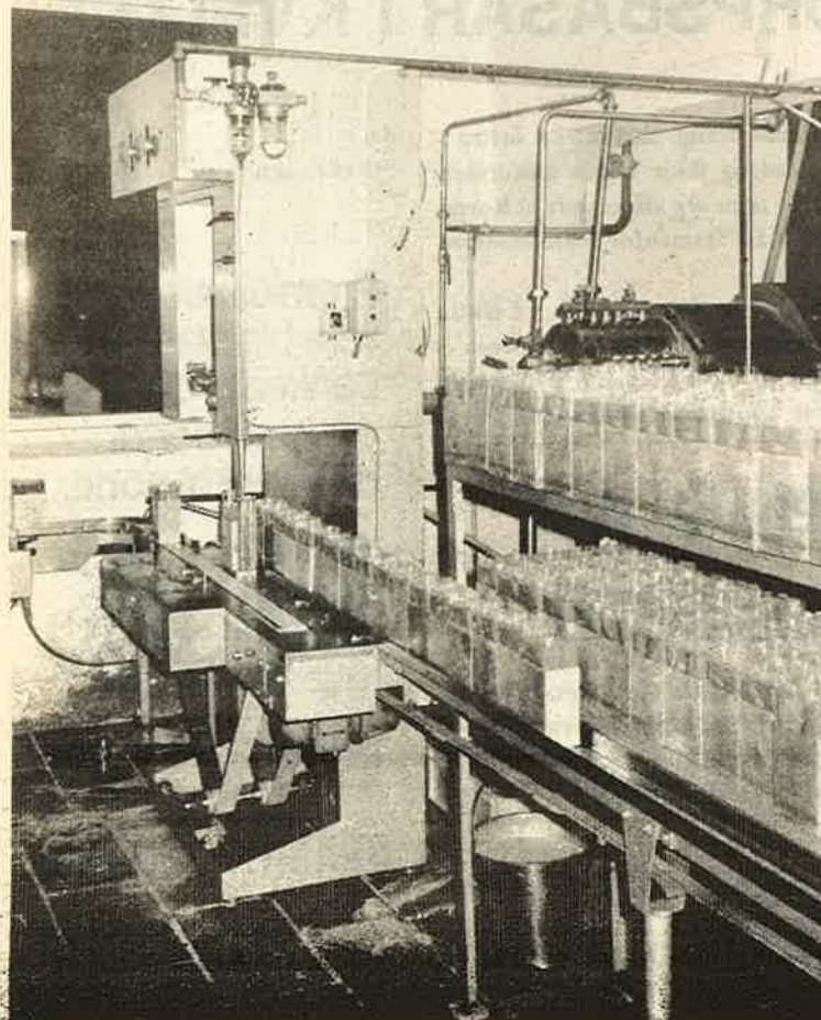
På biletet over står Jon J Tryggestad ved ei av brunostgrytene. På biletet under deler av pakkeanlegget for brunost.
